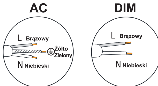
Schemat przyłączeniowy
